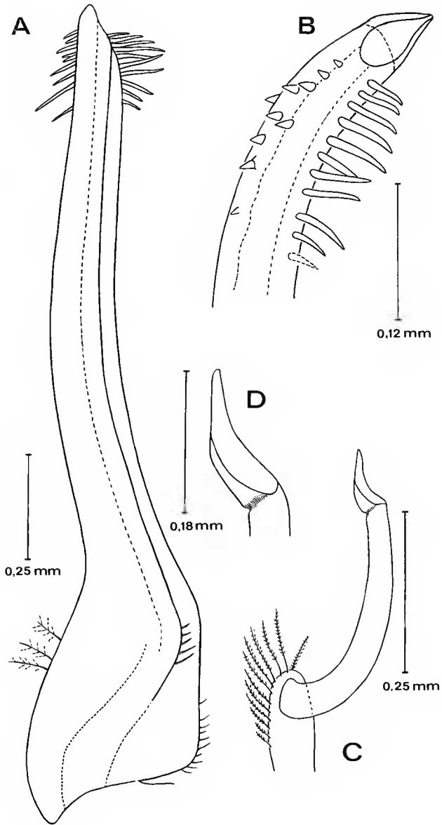
FIG. 6. — Pléopodes sexuels mâles 1 et 2 chez Coralliope armstrongi (Garth), holotype, ♂ 3,1 × 4,5 mm, Ecuador, La Plata Island (AMNH 10010) : A, P11 en entier ; B, id. , apex ; C, P12 en entier ; D, id. , flagelle. (D'après des dessins originaux de J. S. GARTH et non publiés.)
